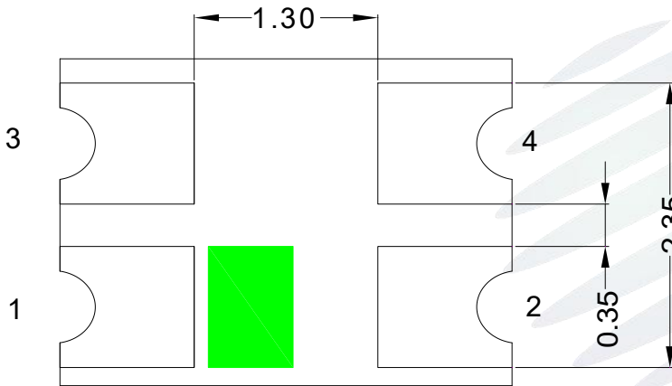
Fig.1-3 Bottom view 背面视图
