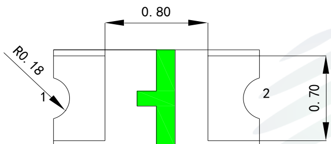
Fig.1-3 Bottom view 背面视图
