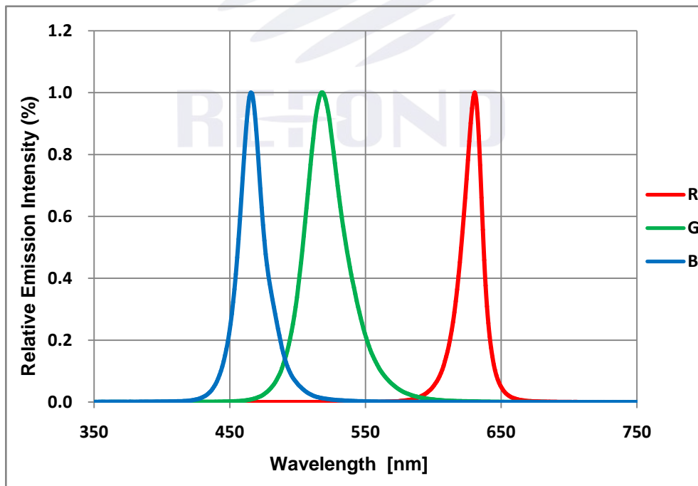
Fig. 1-14 Spectrum Distribution光谱分布特性曲线
