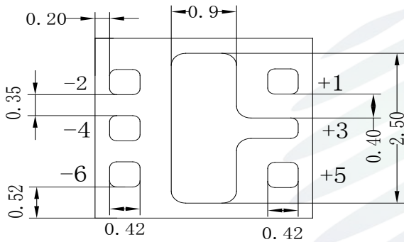
Fig. 1-3 Bottom view 背面视图
