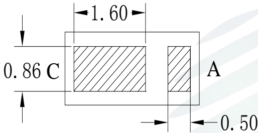
Fig. 1-3 Bottom View 背面视图
