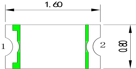
Fig.1-1 Top view 正面视图
