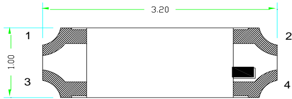
正面视图
