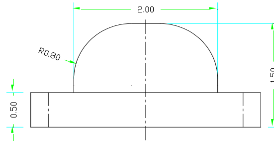
侧面视图
