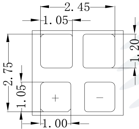
Fig.1-3 Bottom View 背面视图
